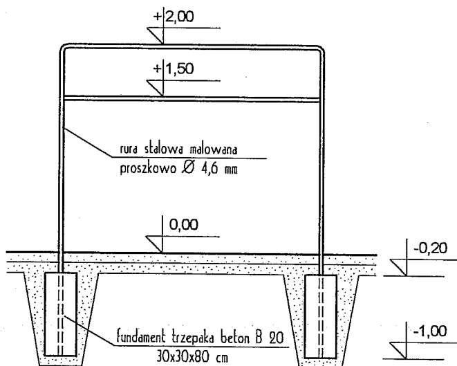
PRZEKRÓJ TRZEPAKA
